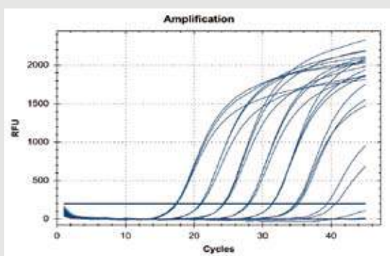
使用例：デングウイルス合成 RNA を使用した Standard Curve の作製
